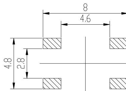
安装尺寸
